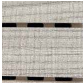
PANNEAU DE BOIS DE MÉLAMINIUM B;S2,dO / COUCHE DE BOIS 14 MM D'ÉPAISSEUR TROUS ARRIÈRE 16X32 FRAISAGE 32-3. TISSU NOIR INSONORISANT À L'ARRIÈRE.
